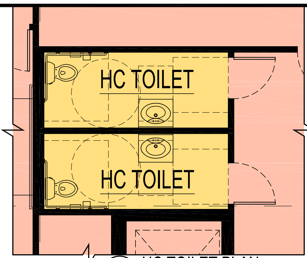
C HC TOILET PLAN A1.4 SCALE: 1/4" = 1'-0"
